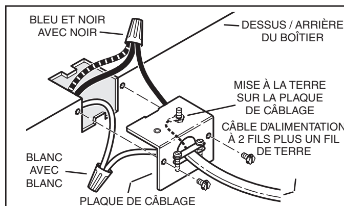
Ventilateur et éclairage commandés par un seul interrupteur
